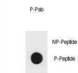
Dot Blot
